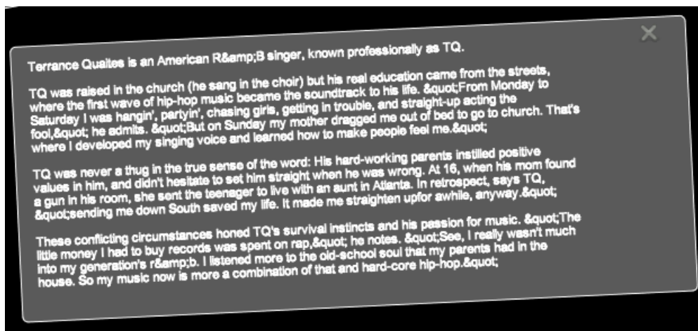
Figuur 1: ArtistInfo
